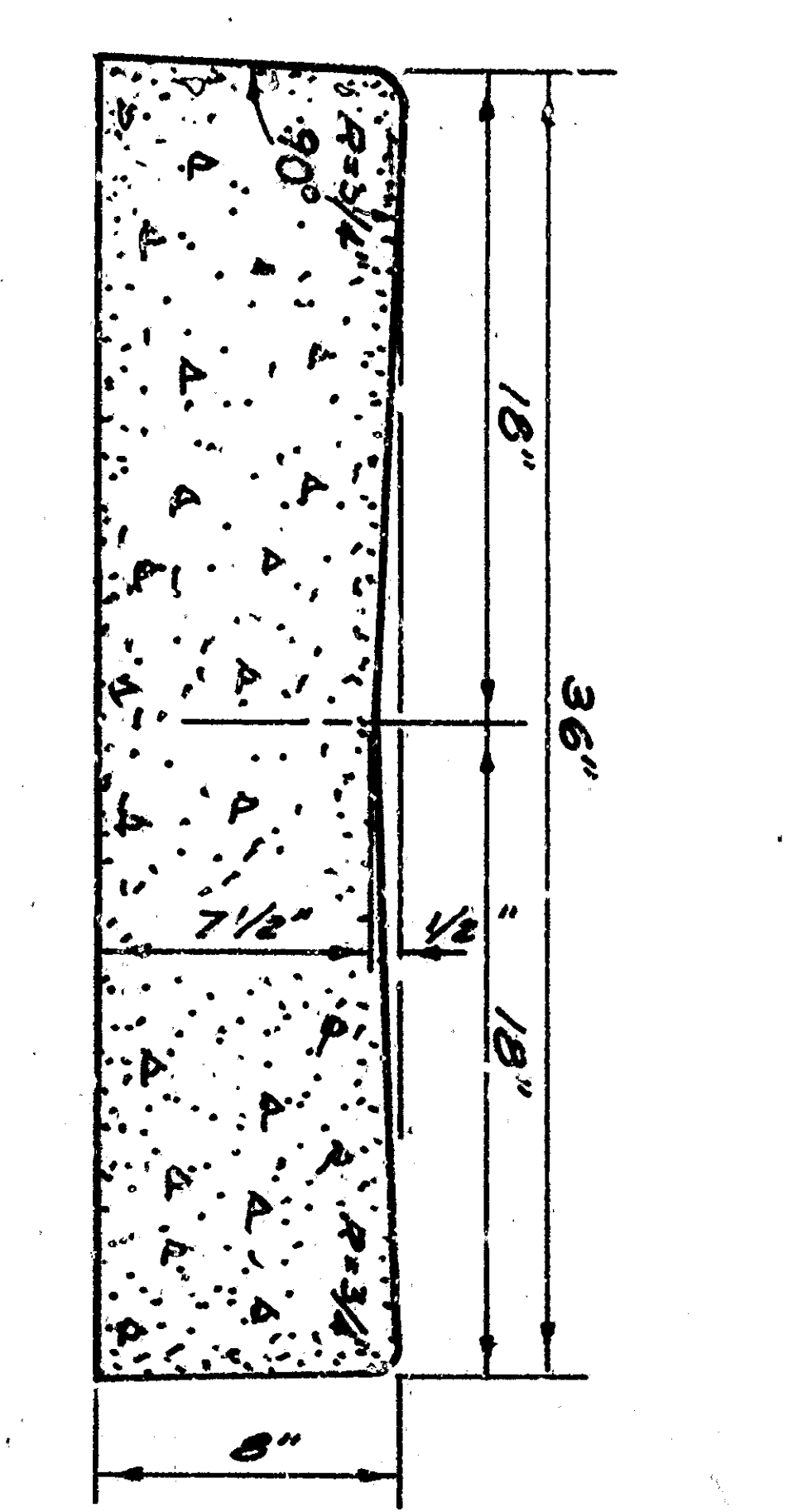
P.C.C. CROSS GUTTER
