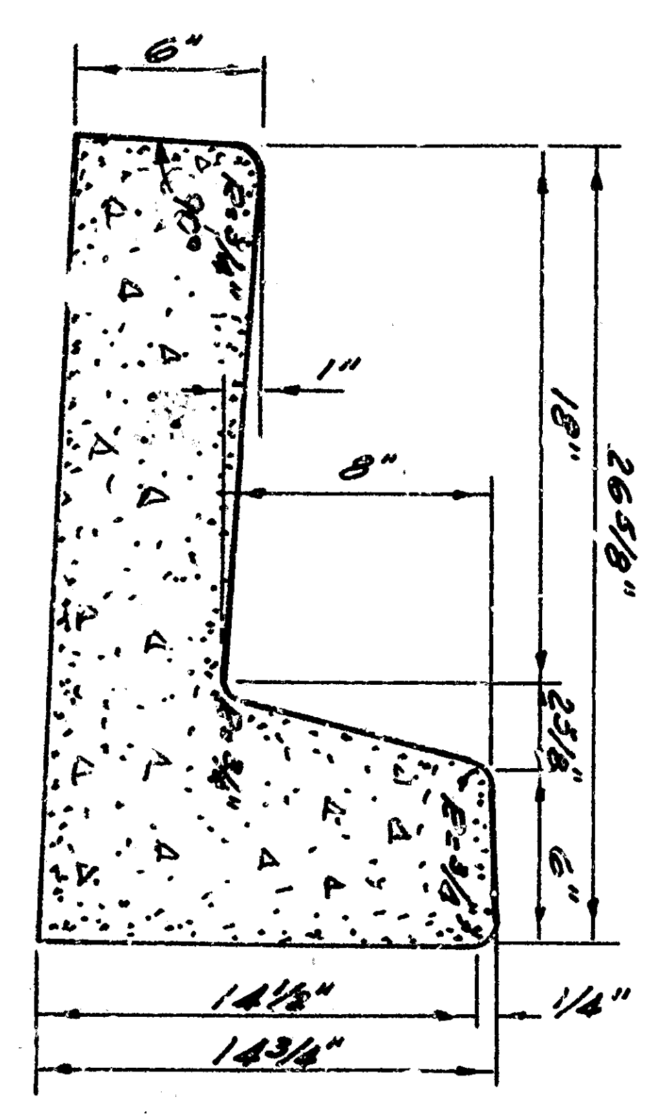
P.C.C. CURB & GUTTER
